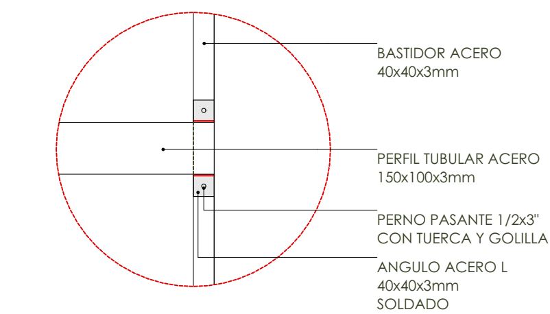
D01 | DETALLE UNIÓN ESTRUCTURA Y BASTIDOR 1:10
