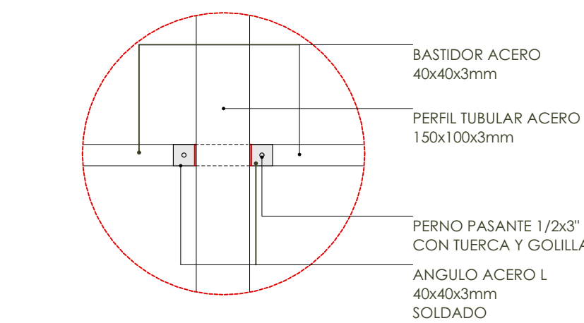
D02 | DETALLE UNIÓN ESTRUCTURA Y BASTIDOR 1:10
