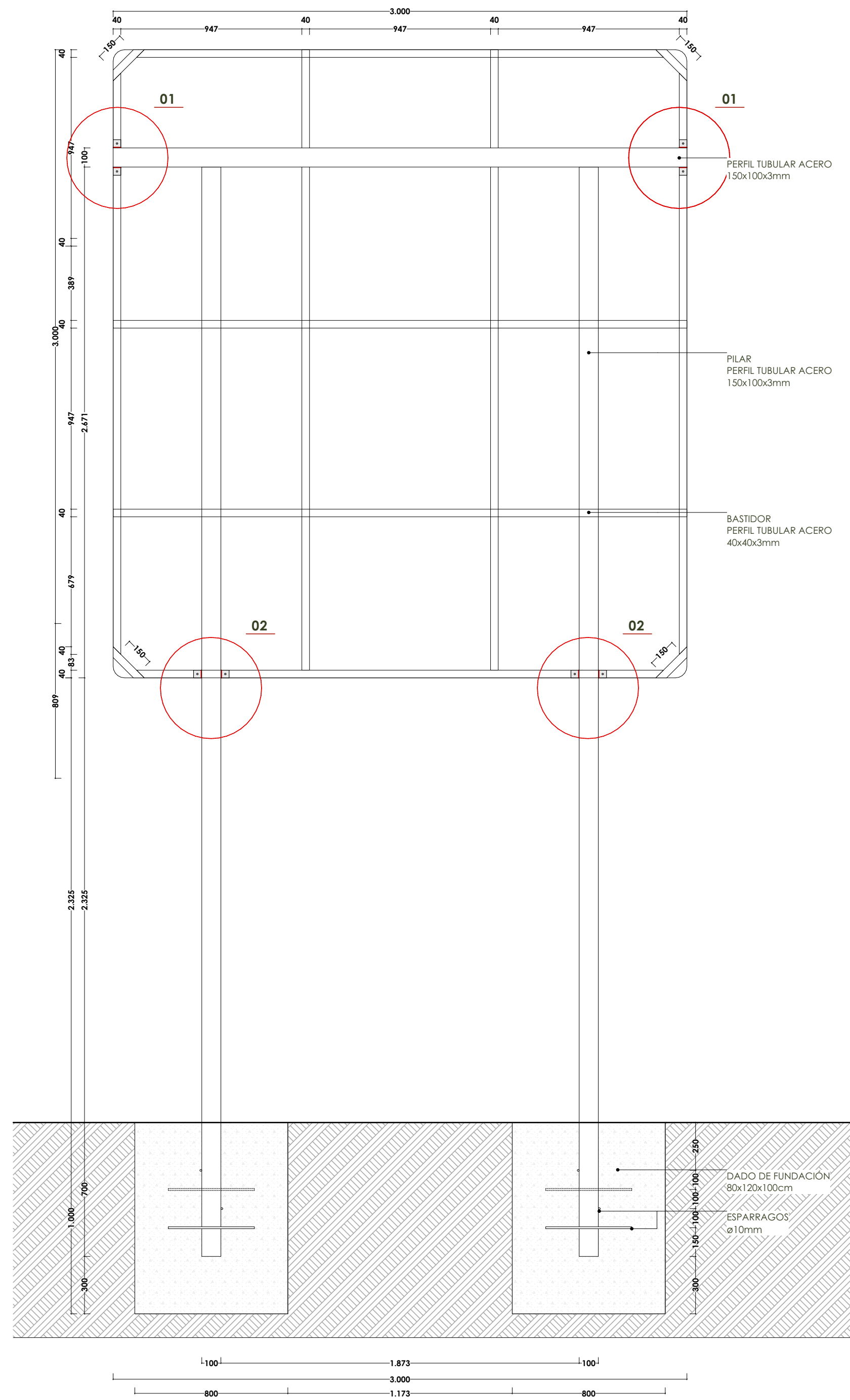
E01 | ELEVACIÓN POSTERIOR 1:20
