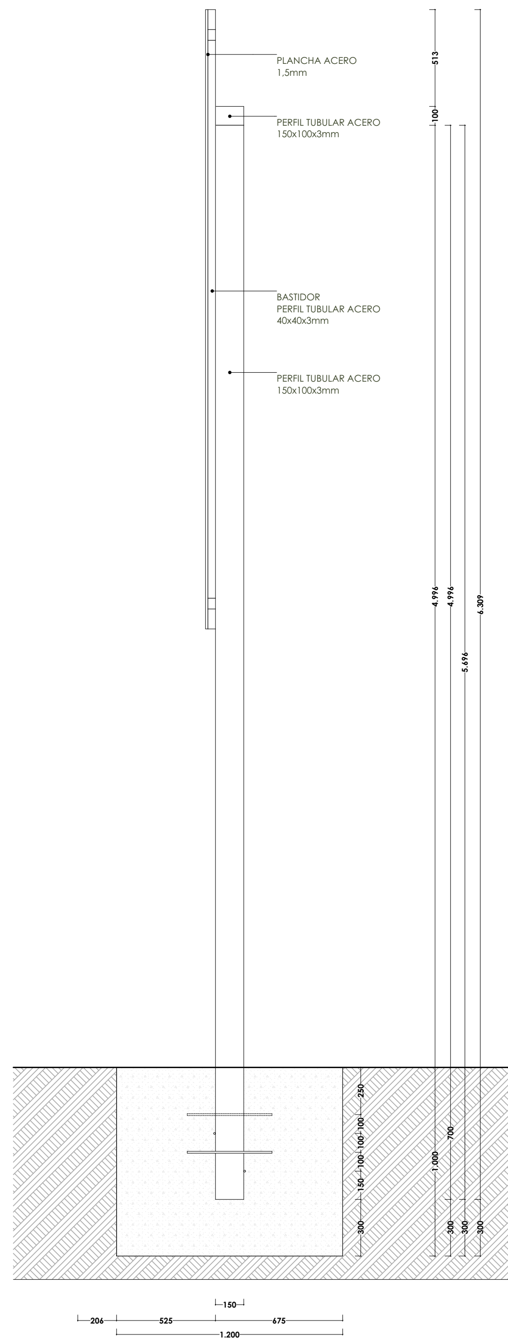
E01 | ELEVACIÓN LATERAL 1:20
